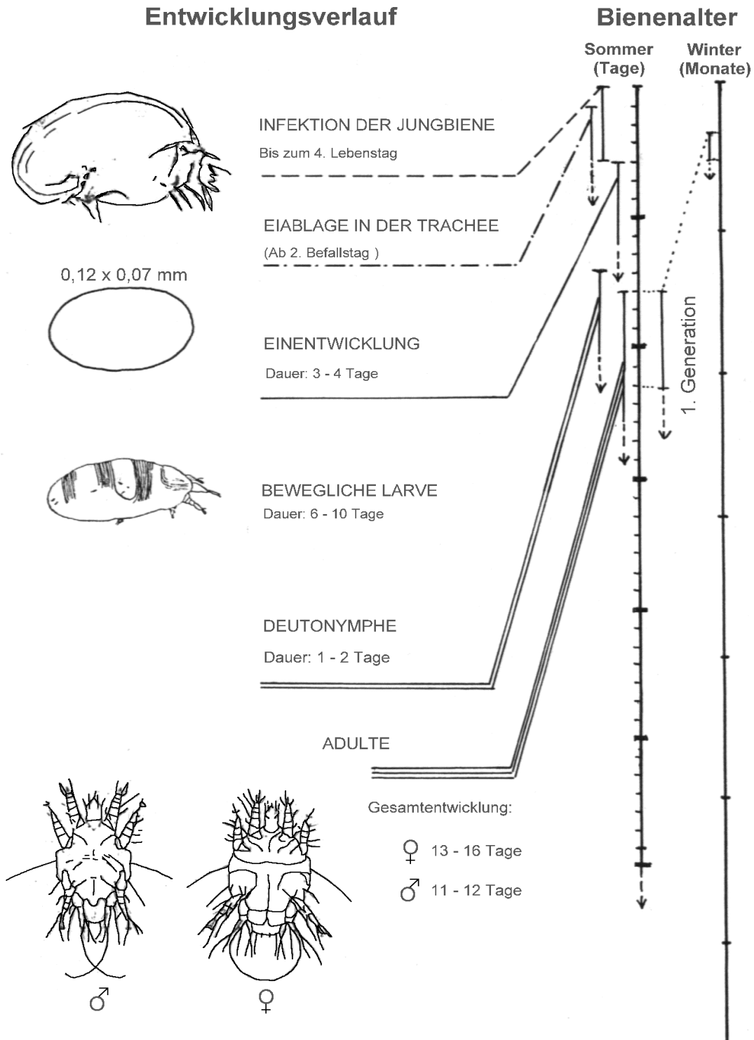
Abb. 1 – Entwicklungslauf von Tracheenmilbe und Biene
